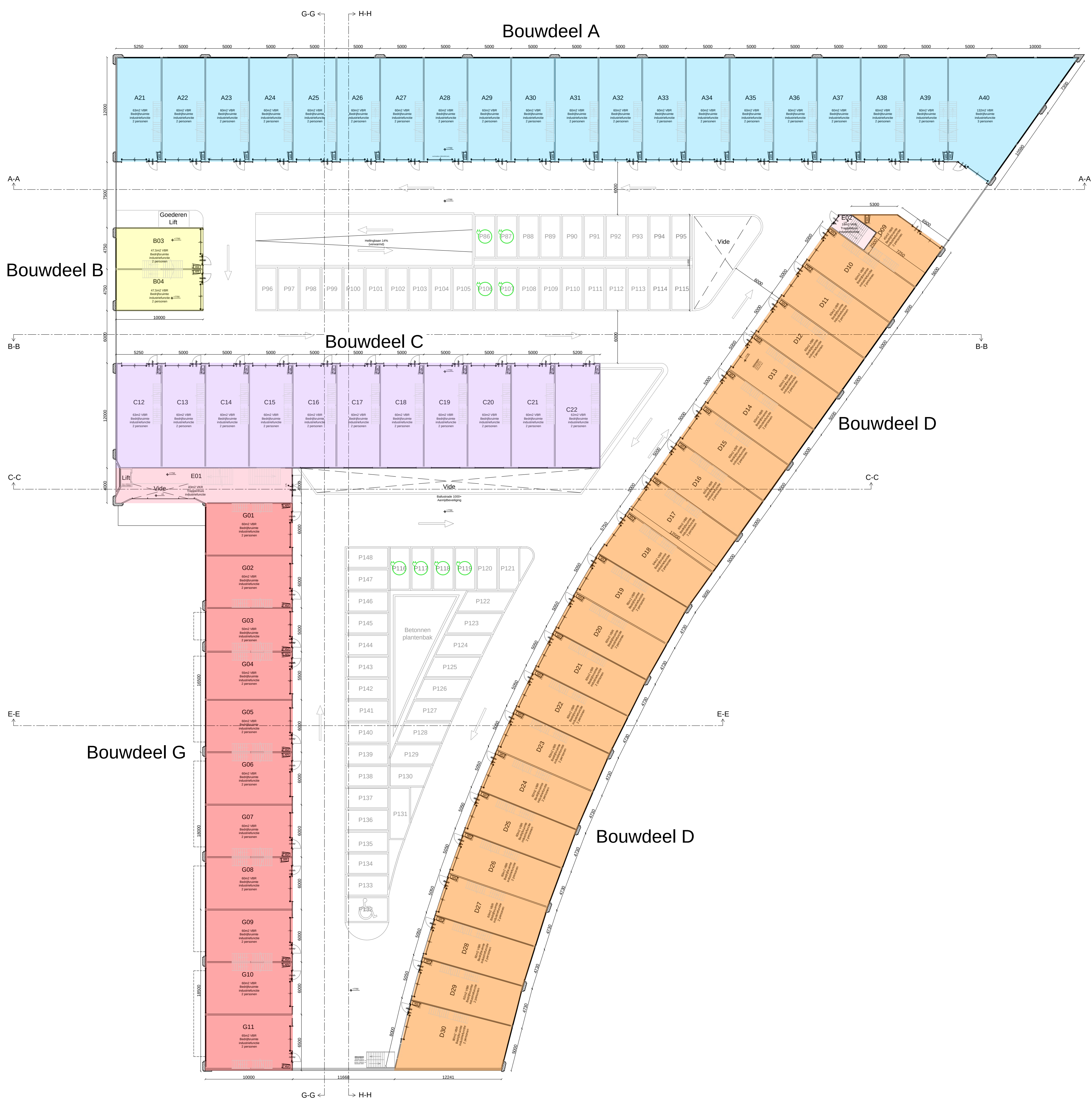
Plattegrond 2e verdieping (deknivo)
