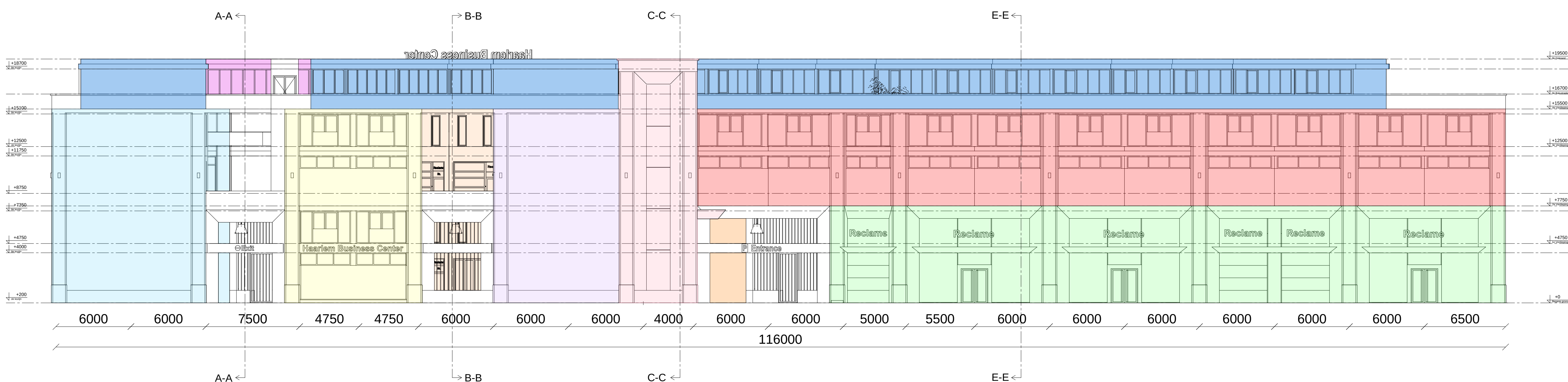
Zuidgevel (Kuipersweg zijde)
