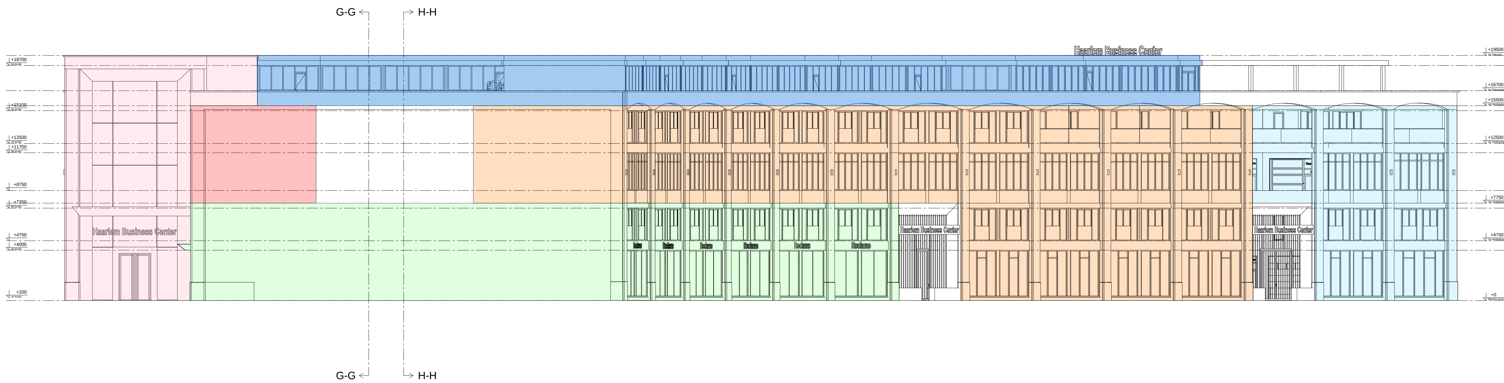
Oostgevel
