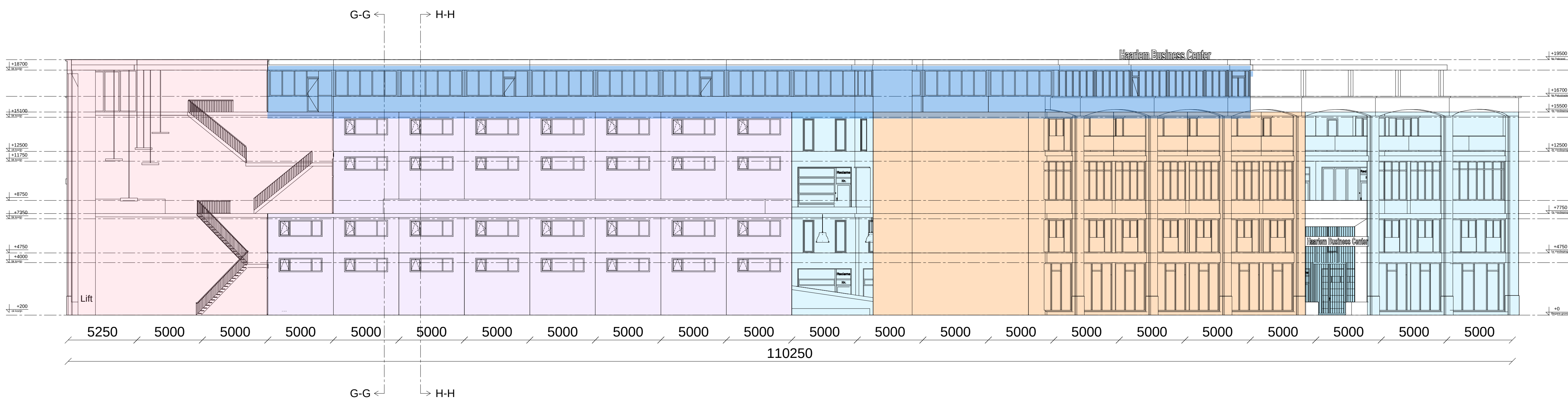
Doorsnede C-C
