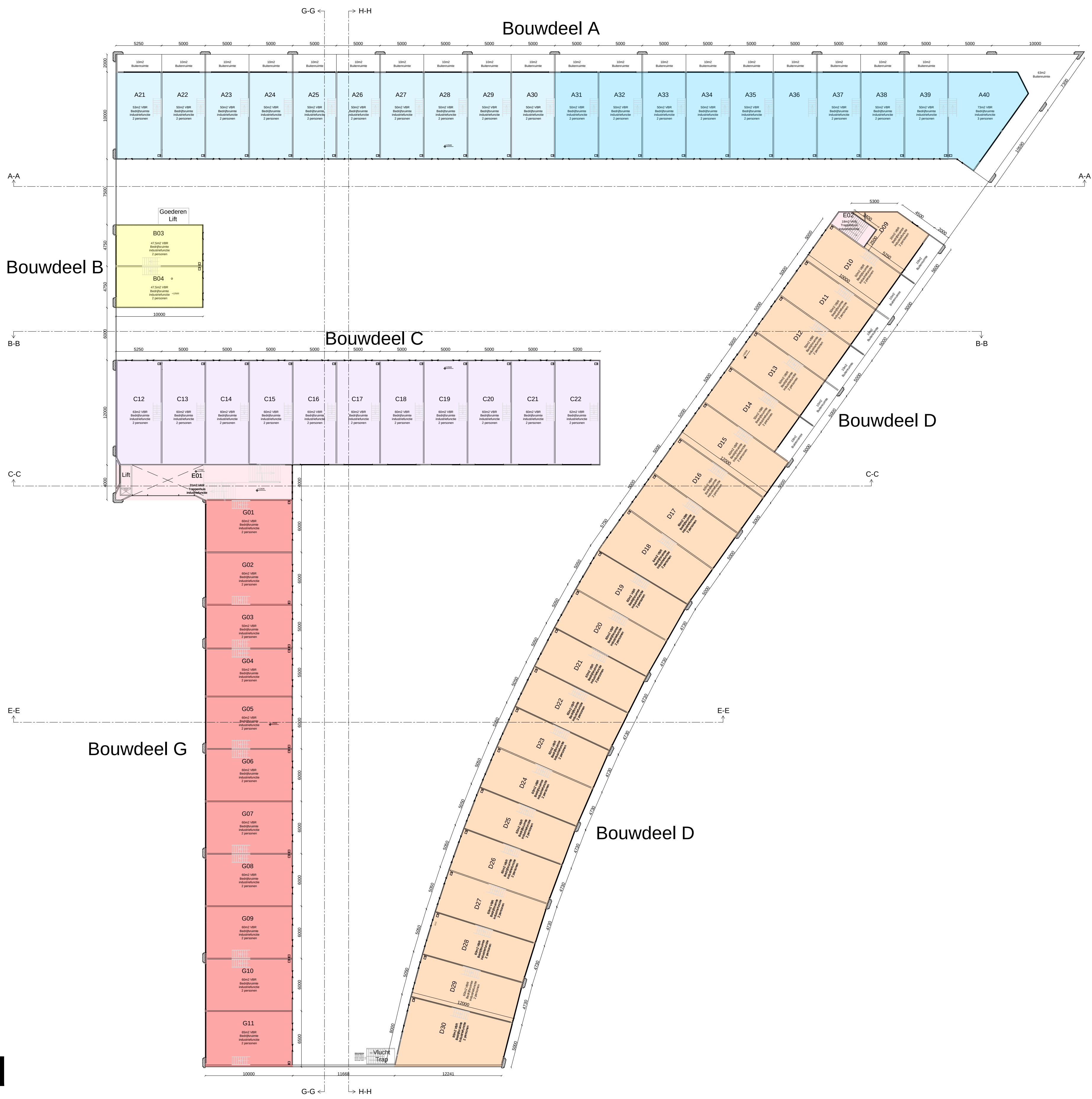
Plattegrond 3e verdieping (deknivo)
