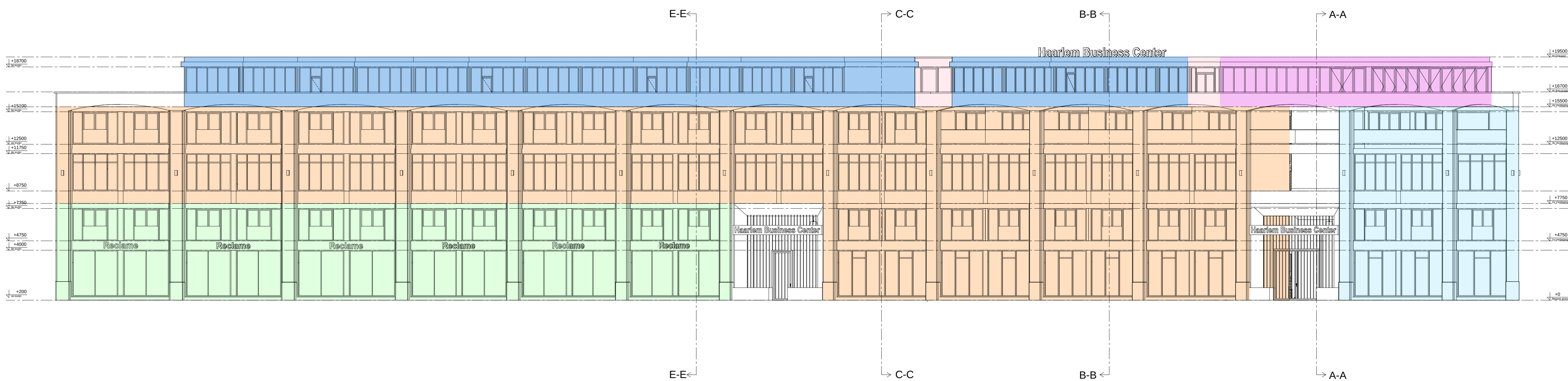
Noordgevel (Waarderweg zijde)
