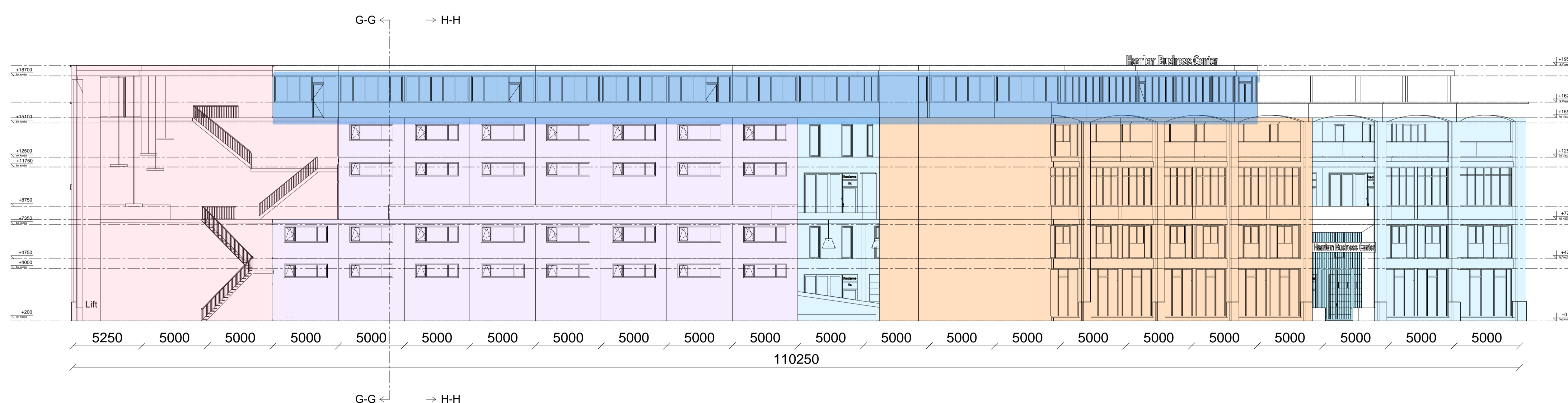
Doorsnede C-C
