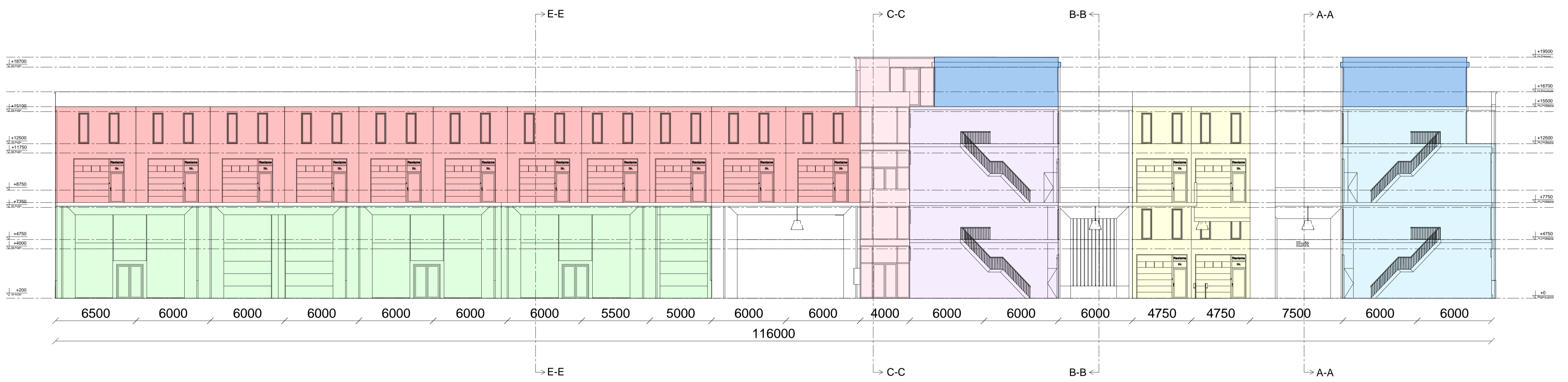
Doorsnede G-G
