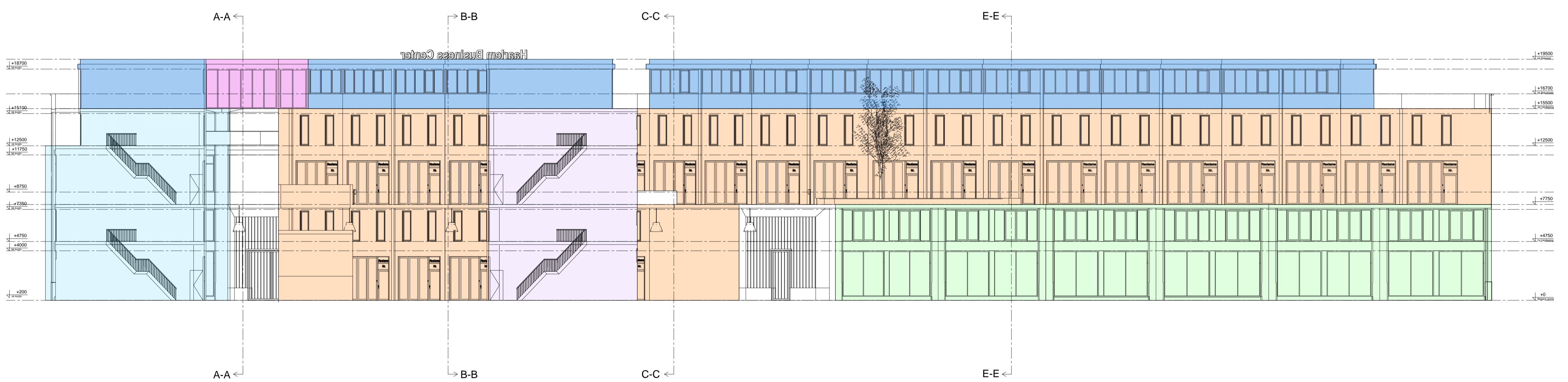
Doorsnede H-H
